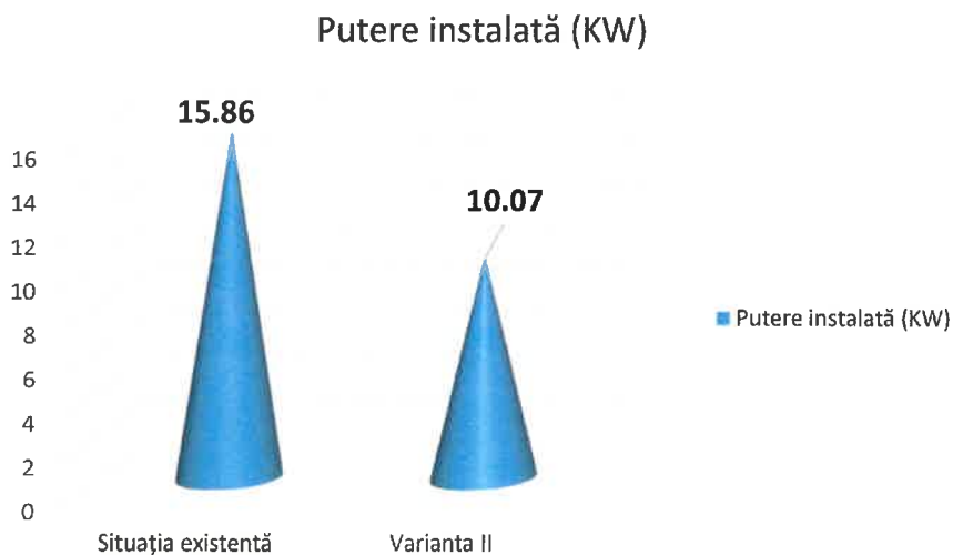
Fig. 14 Comparăție putere totală instalată
